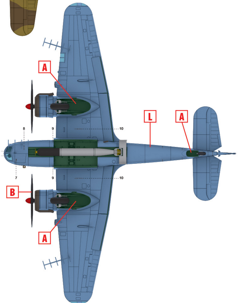
4) Bristol Beaufort Mk.IA EK979, навчальний підрозділ RAF, Більбейс, Єгипет, 1944 рік Bristol Beaufort Mk.IA EK979, RAF training unit, Bilbais, Egypt, 1944
